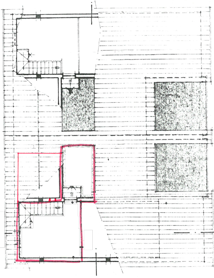
PIANTA PIANO SOTTOTERRITTO - COPERTURA
