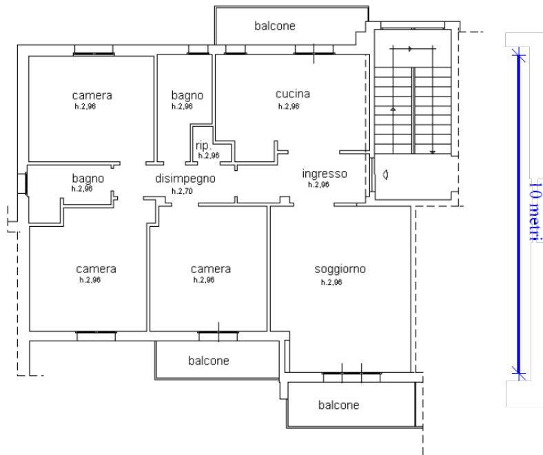
PIANO PRIMO
