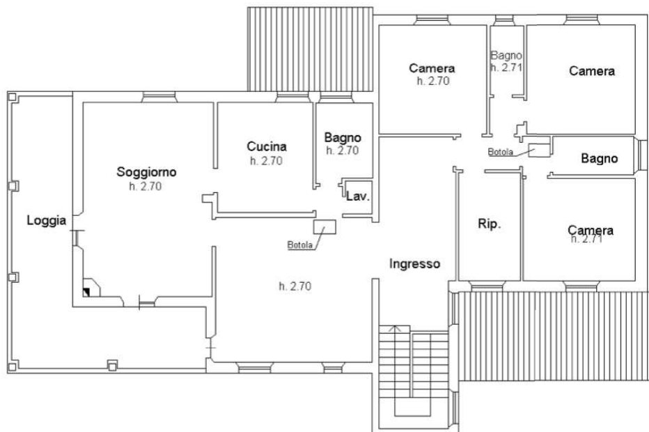
PIANO PRIMO
