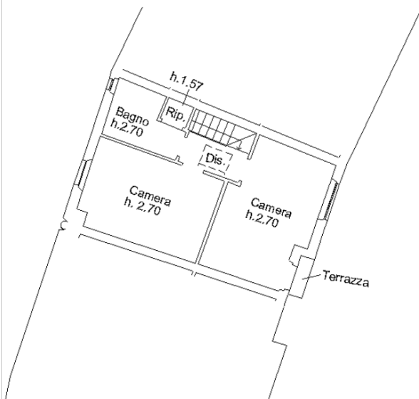
PIANO PRIMO
