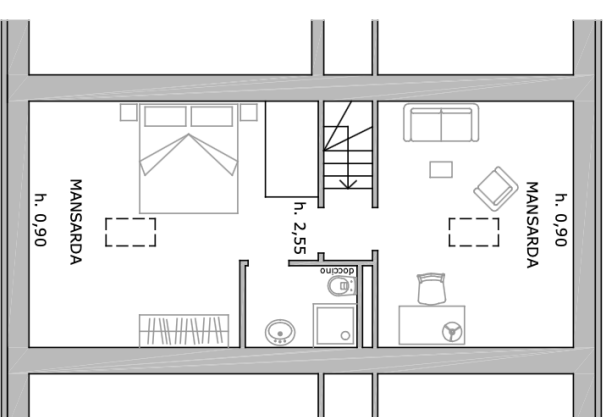
PIANO SECONDO (mansarda)
