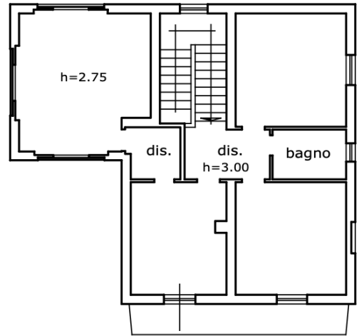
PIANO 1°
