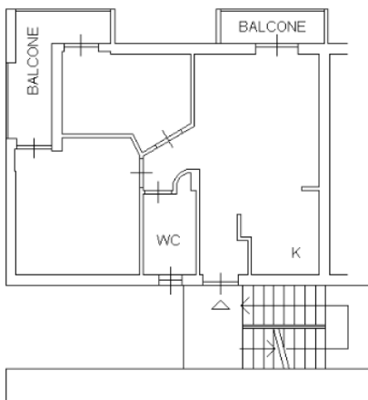
PIANO PRIMO (H = 2,70 mt)
